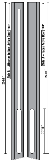
Left Hand T-Astragal
